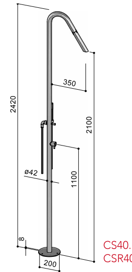
CS40 CSR40
